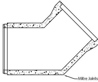
Single Mitre Bend
