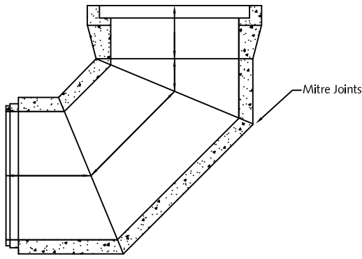
Double Mitre Bend
