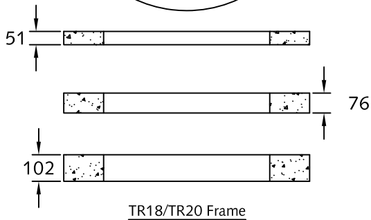
TR18/TR20 Frame
