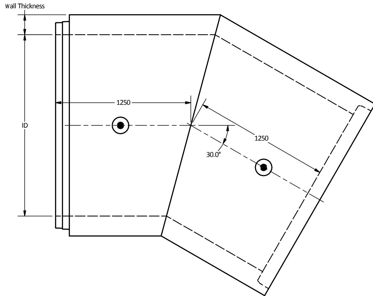
Single Mitre Bend (30°)
